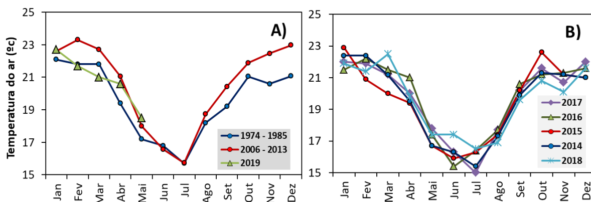
Figura 2: Temperaturas médias do ar (°C) das médias históricas de 1974-1985, 2006-2013 e 2019 (A) e dos anos de 2014, 2015, 2016, 2017 e 2018 (B) para a região do Sul de Minas, Muzambinho.
