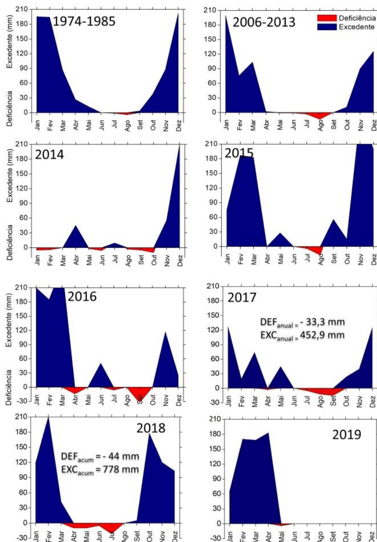
Figura 8: Balanço hídrico mensal sequencial (THORNTHWAIT E MATHER, 1955) no período de 1974-1985 (A), 2006-2013 (B), para os anos de 2014 (C), 2015 (D), 2016 (E), 2017 (F), 2018 e 2019 para a região do Sul de Minas, Muzambinho.
